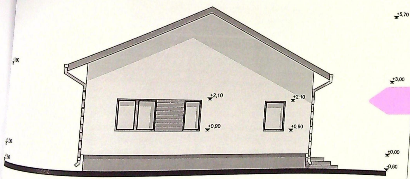
FATADA NORD
