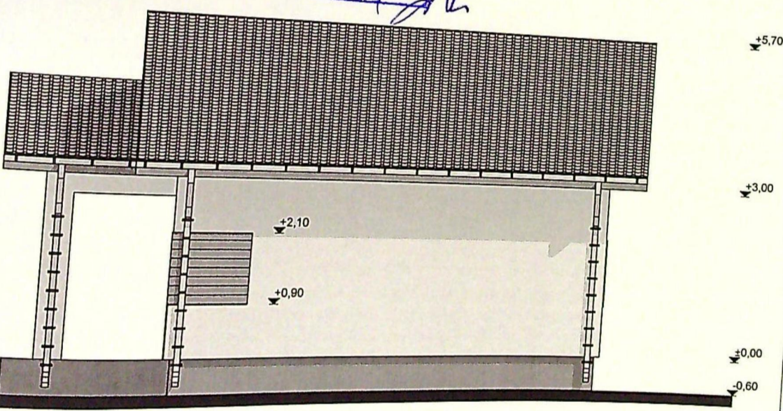
FATADA EST
